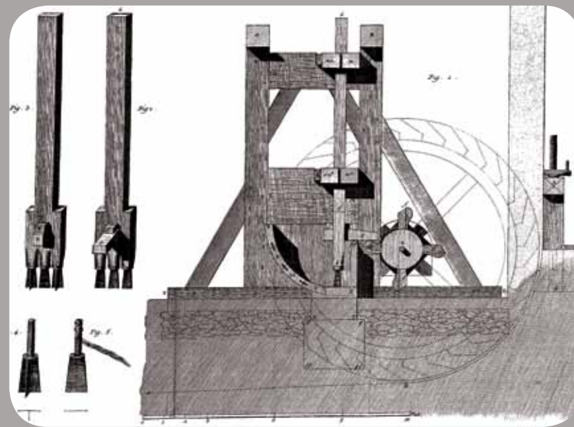
Schéma d'un moulin à tan, coupe transversale © Encyclopédie des sciences, des arts et des métiers
