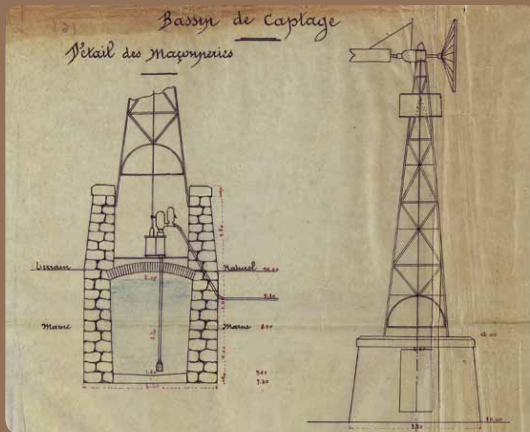
Détail des maçonneries, projet de l'éolienne, 1927 © Archives Départementales de l'Ariège 201246
