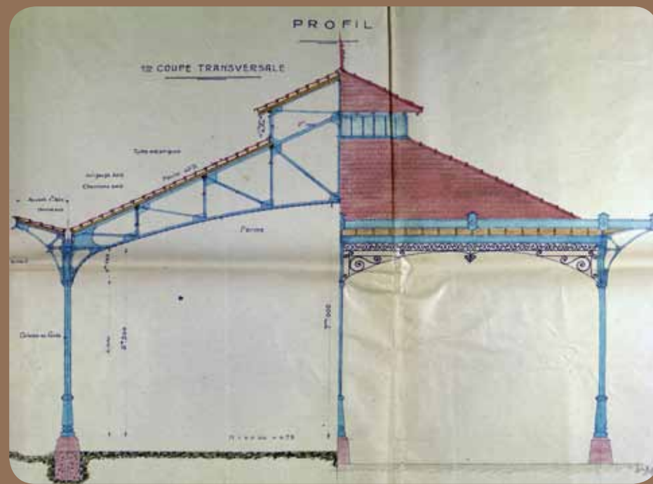
Projet de halle non exécuté © Archives Départementales de l'Ariège 70EDTIM2
